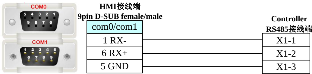
RS485-2 通讯电缆
