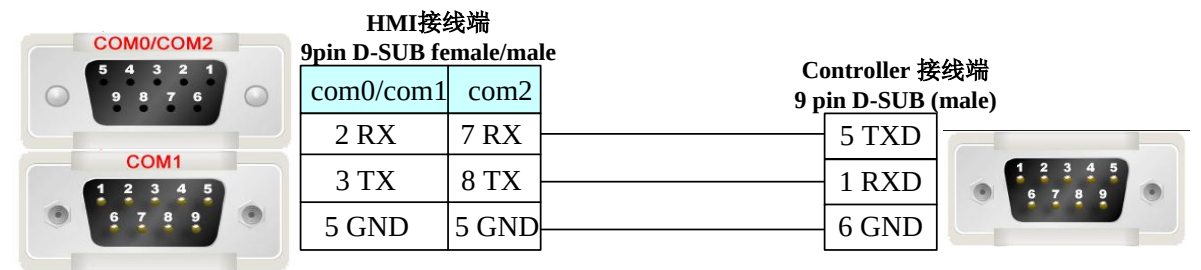
RS232 通讯电缆
