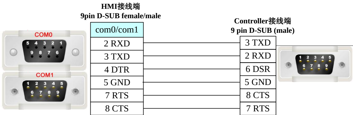
RS232 通讯电缆
