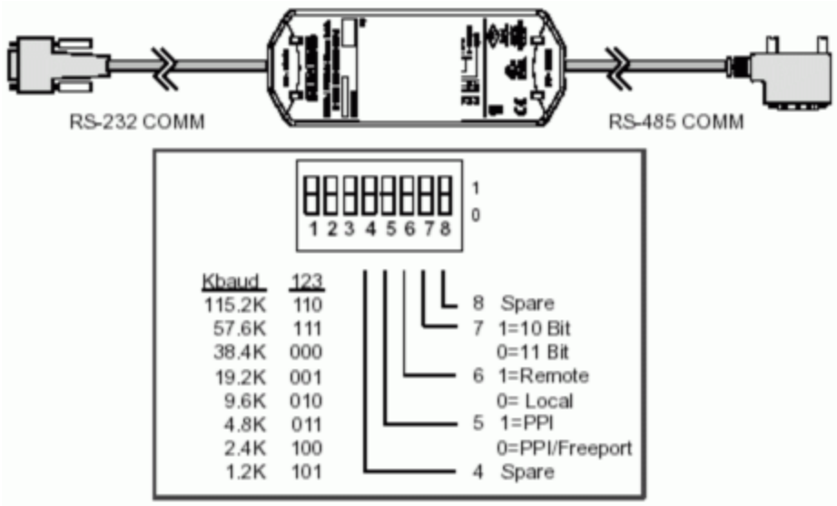
PC/PPI 电缆波特率开关选择
