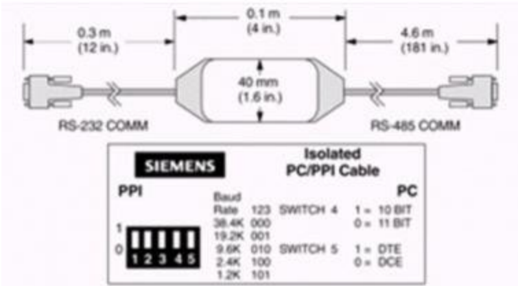
PC/PPI 电缆波特率开关选择
