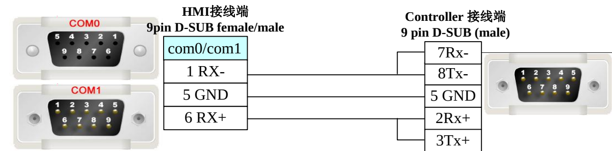
RS485-2 通讯电缆
